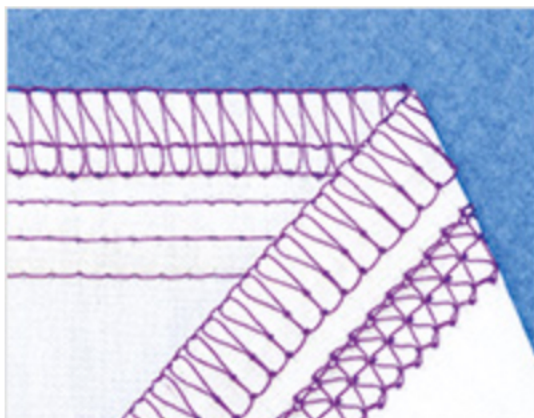
4-ниточный оверлочный и тройной закрывающий шов
